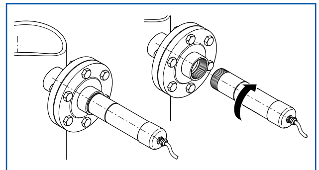
Abb. 4: Flanschmontage
