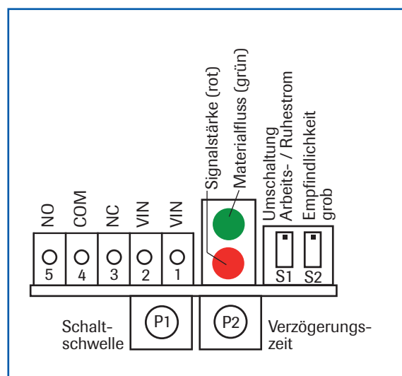
Abb. 11: Lage der Bedienelemente
