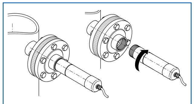
Abb. 6: Montage mit Trennflansch
