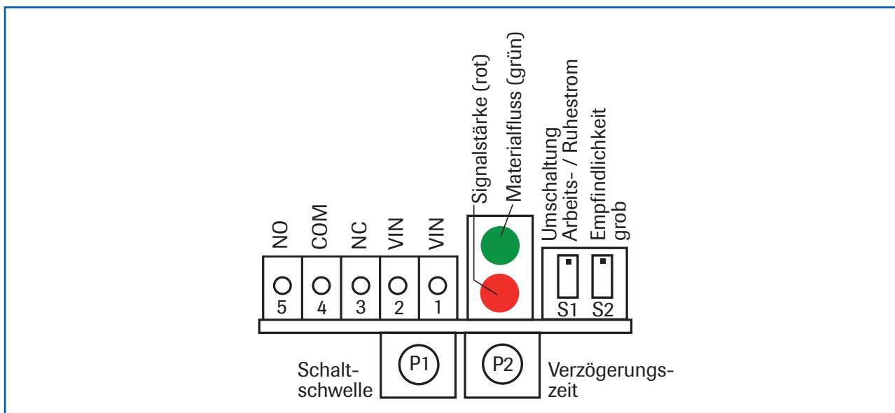
Abb. 9: Anschluss- und Bedienelemente
