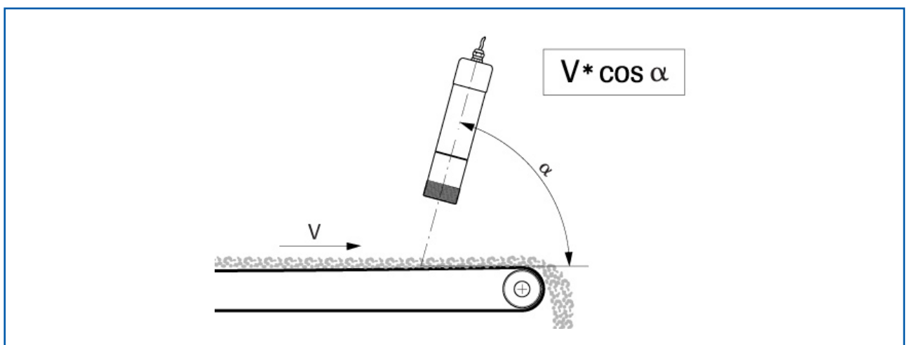
Abb. 8: Ermittlung des Anstellwinkels
