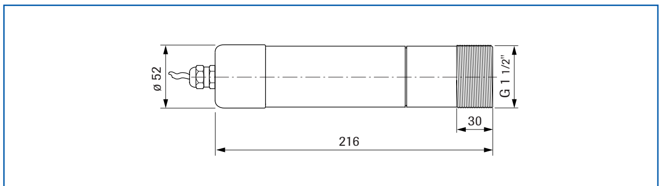
Abb. 2: Maßzeichnung
