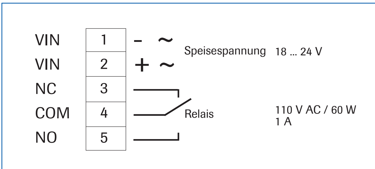
Abb. 10: Anschlussbild Sensor
